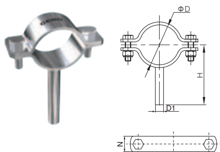
TH5-A Tubing Hanger
