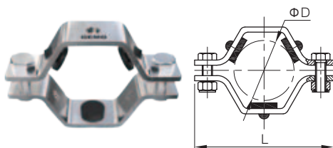
TH4-A Tubing Hanger
