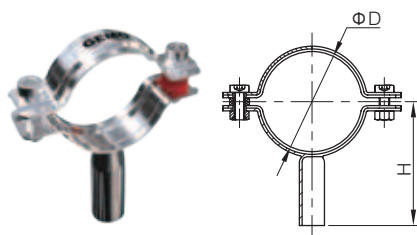
TH2 Tubing Hanger
