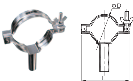
TH1-A Tubing Hanger
