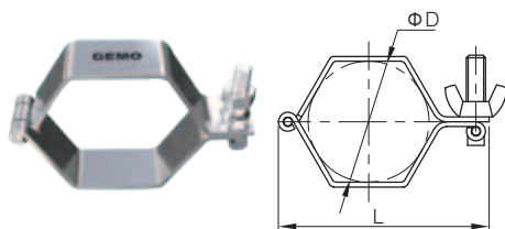
TH3-A Tubing Hanger
