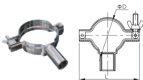
TH1-B Tubing Hanger
